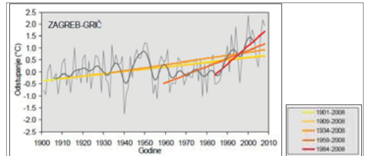
Slika 2. Vremenski nizovi srednje godišnje temperature zraka, pripadni 11-godišnji binomni klizni srednjaci i trendovi za 108-, 100-, 75-, 50- i 25-godišnje razdoblje (jedinice su odstupanja (°C) od srednjaka 1961.-1990.)
